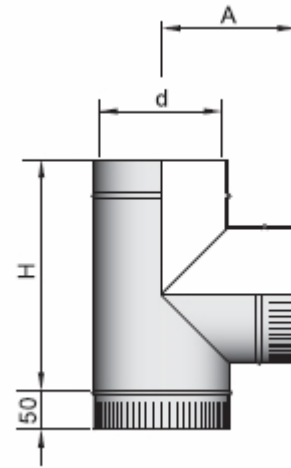
Тройник TRH 90°
