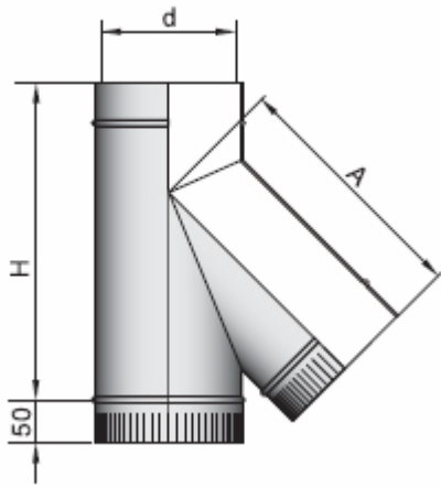
Тройник TRH 45°
